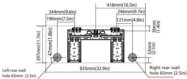
MSAGBU-09 y MSAGBU-12
