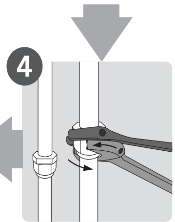
4 Conectar las tuberías de refrigerante.
