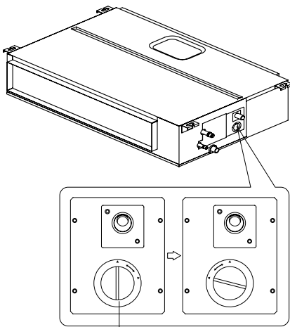
Tapa de prueba
