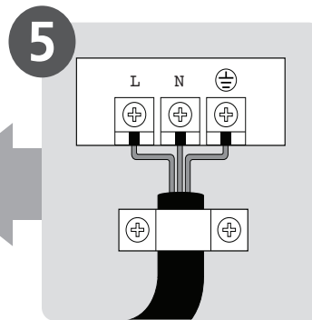
5 Conectar los cables
