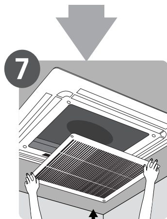
7 Instalar el panel frontal
