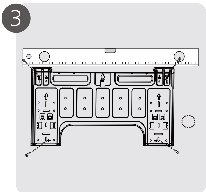
Colocar la placa de montaje
