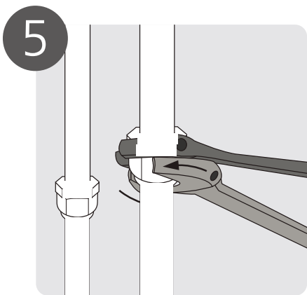
Conecte la tubería
