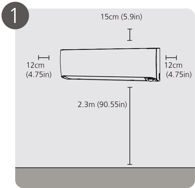
Seleccione la ubicación de la instalación
