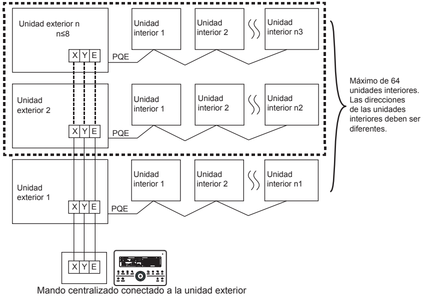
Mando centralizado conectado a la unidad exterior
