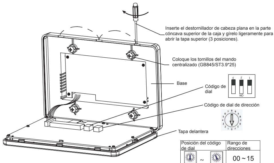
Fig. 1.2 Diagrama de instalación
