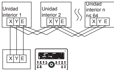
Mando centralizado conectado a la unidad interior
