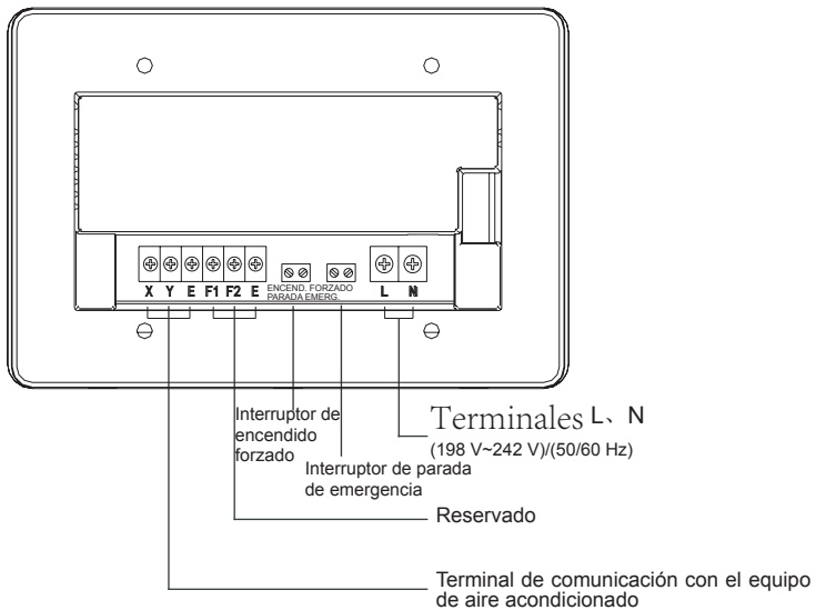
Fig. 1.3 Instrucciones del terminal del mando centralizado
