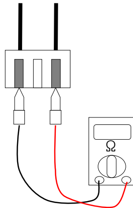
<Tipo Cassette (1 vía, 4 vías) / Tipo conducto oculto en el techo >
