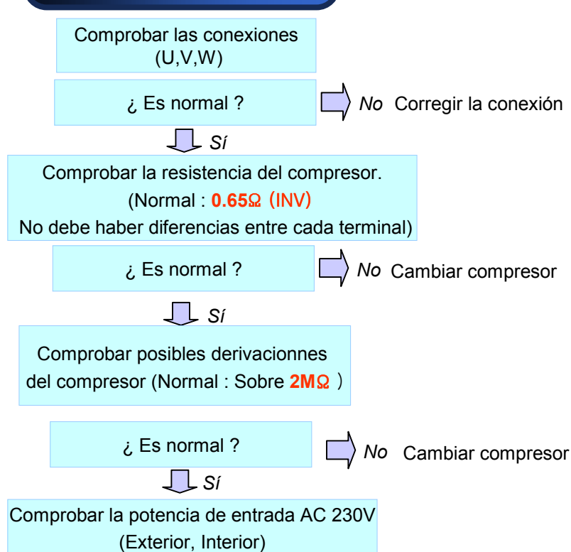
Compresor
