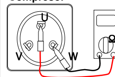
Compresor
